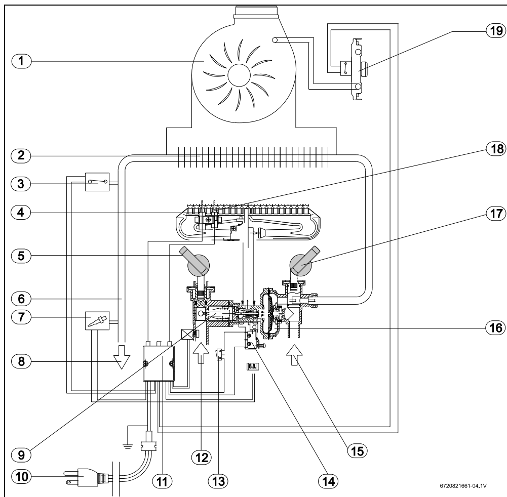
Fig. 2 Esquema técnico
