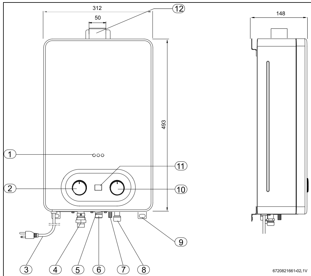
Fig. 1 Dimensiones
