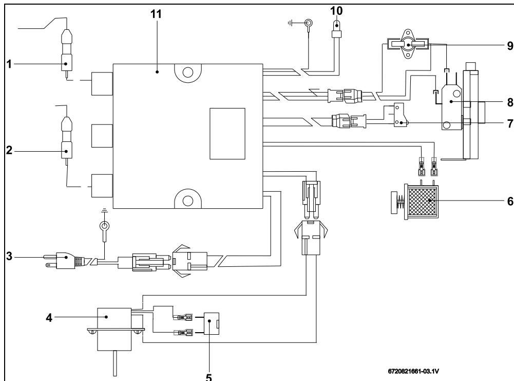
Fig. 3 Esquema eléctrico
